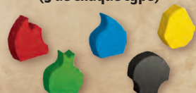
25 pions Essence (5 de chaque type)
